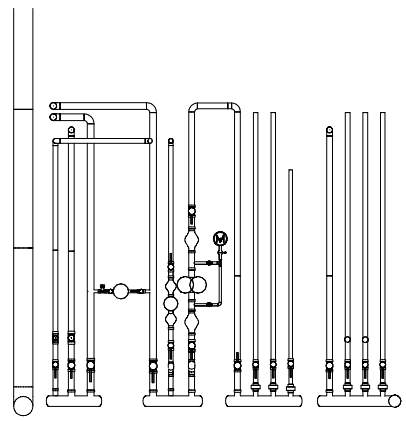
SEZ. A-A (1:20)
